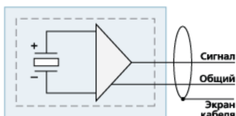
Рис. 1.3 Структурная схема гидрофонов ВС 312
